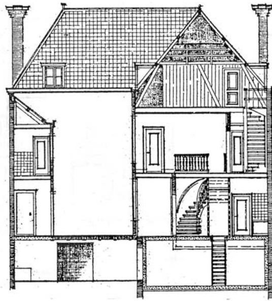
doorsnede CD
